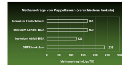
Abb. 2: Methanerträge von Pappelholzfasern
