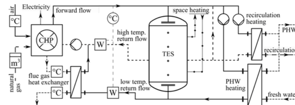
Abb. 1: Reduziertes Funktionsschema des Feldtests mit BHKW, Speicher und TWE-Anlage
