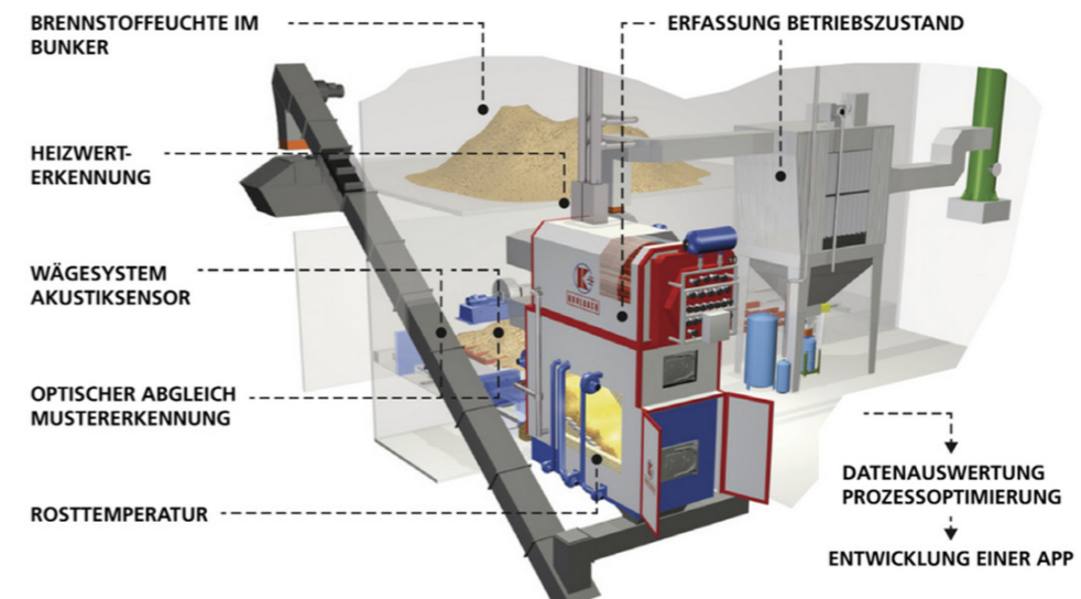
Abb. 1: Entwicklung innovativer Sensorik für Biomassefeuerungen im Rahmen des Projekts DigitalFire (Quelle: ©Kohlbach/Fraunhofer/Umsicht)
