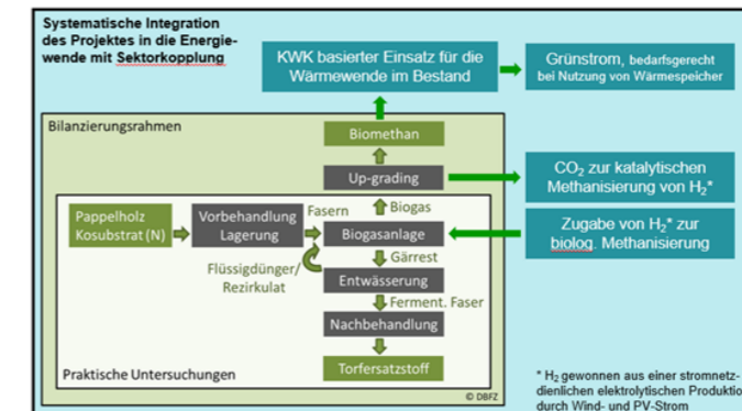
Abb. 1: Darstellung des Untersuchungs- und Bilanzrahmens sowie der Integration des Projektes in die Energiewende
