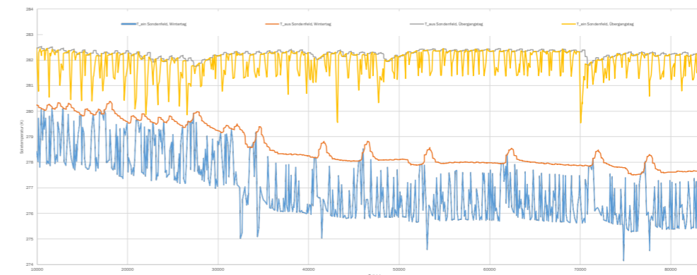
Abb. 1: Temperaturverläufe der Sole im Wärmenetz vor und nach Durchströmung des Sondenfeldes für zwei Typtage.
