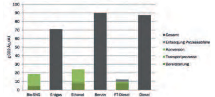
Abbildung 22: Treibhausgasbilanzen für strohbasierende Kraftstoffkonzepte (Äq.: Äquivalente, FT: Fischer Tropsch, MJ: Megajoule, SNG: Synthetic Natural Gas)
