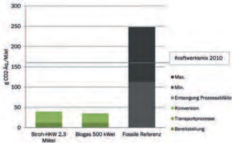
Abbildung 21: Treibhausgasbilanzen für strohbasierende KWK-Konzepte (Äq.: Äquivalente, el: elektrisch, FT: Fischer Tropsch, HKW: Heizkraftwerk, kW: Kilowatt, MJ: Megajoule, MW: Megawatt)
