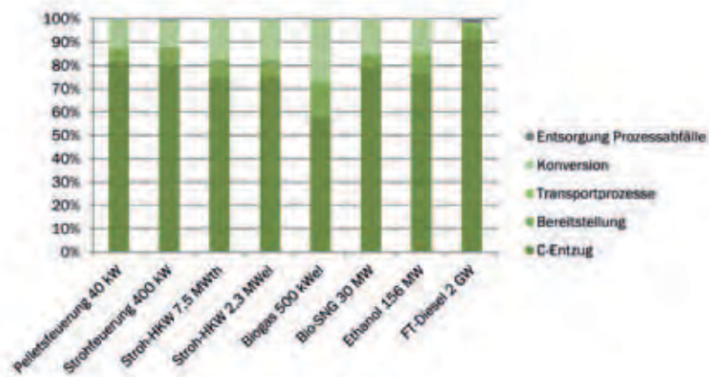
Abbildung 18: Prozentualer Anteil der einzelnen Prozessschritte an den Gesamtemissionen (C: Kohlenstoffzug, el: elektrisch, FT: Fischer Tropsch, GW: Gigawatt, HKW: Heizkraftwerk, kW: Kilowatt, MW: Megawatt, th: thermisch)
