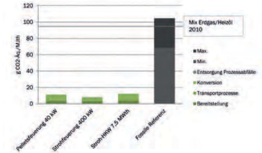
Abbildung 20: Treibhausgasbilanzen für strohbasierte Wärmekonzepte (Äq.: Äquivalente, HKW: Heizkraftwerk, kW: Kilowatt, MJ: Megajoule, MW: Megawatt, th: thermisch)
